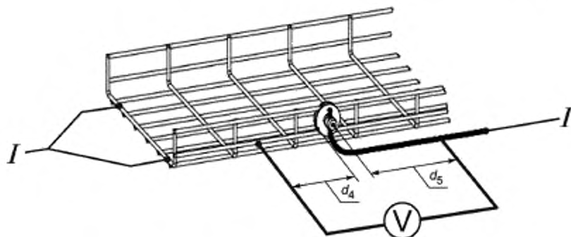
Рисунок 30 — Схема проведения испытания зажимом для присоединения проводника уравнивания потенциалов
