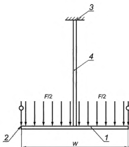
1 — кронштейн с центральной опорой; 2 — точка измерения прогиба на конце кронштейна с центральной опорой; 3 — жесткая конструкция; 4 — подвес; F/2 — нагрузка на кронштейн с каждой стороны подвеса; W — длина кронштейна с центральной опорой
