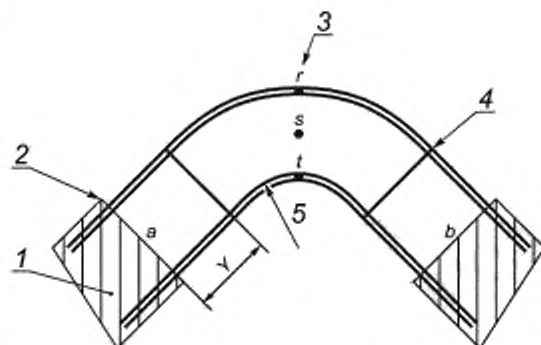
1 — закрепленный участок трассы; 2 — край опоры a или b ; 3 — точки a , s и t измерения прогибов; 4 — типичное положение стыков; 5 — радиус секции; Y — расстояние между опорой и местом соединения секций, заявленное производителем или ответственным лицом, но не более 600 мм
